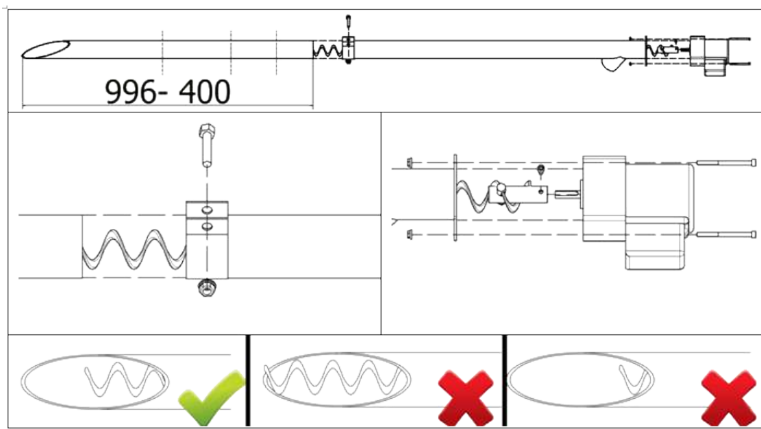
Рисунок 9 – Схема установки винтового подающего устройства в штучере бункера
