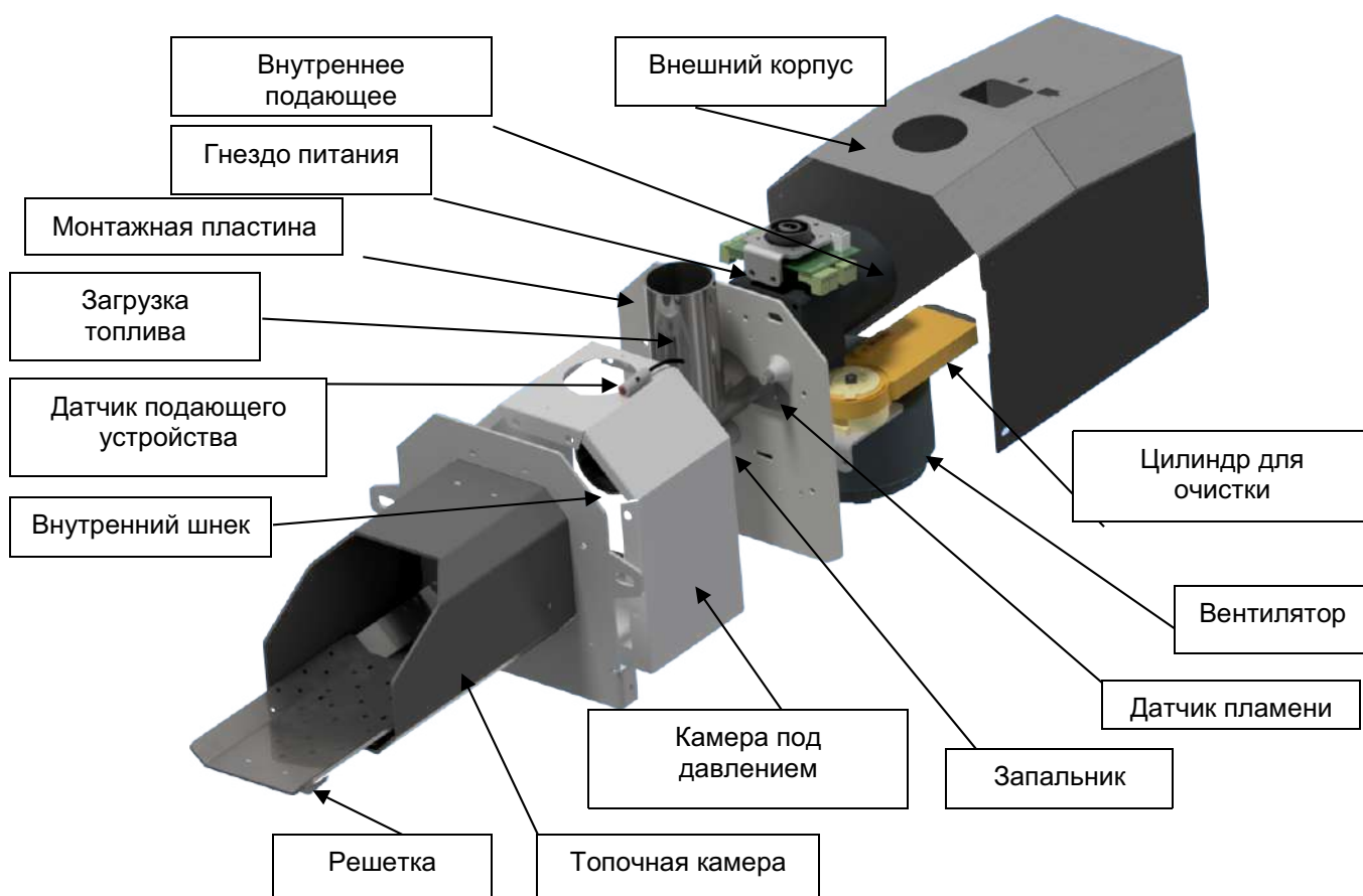
Рисунок 6 – Состав Горелок Lavoга Eco 16-102
