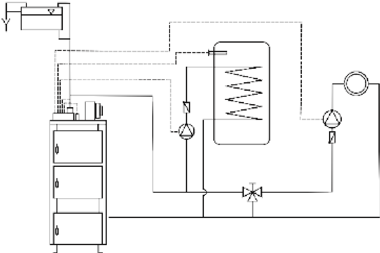
Рисунок 3 - Подключение с трехходовым клапаном и водонагревателем
