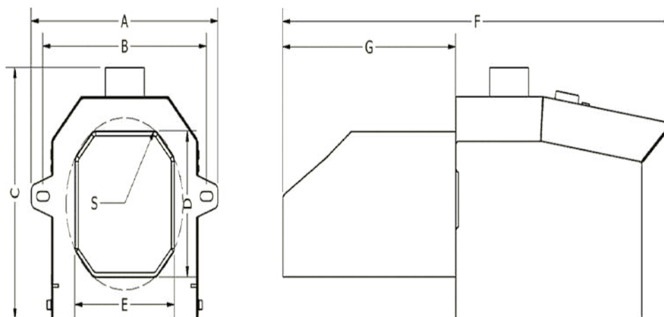
Рисунок 5 – Габаритные и присоединительные размеры Горелок Lavoro Eco 16-102
