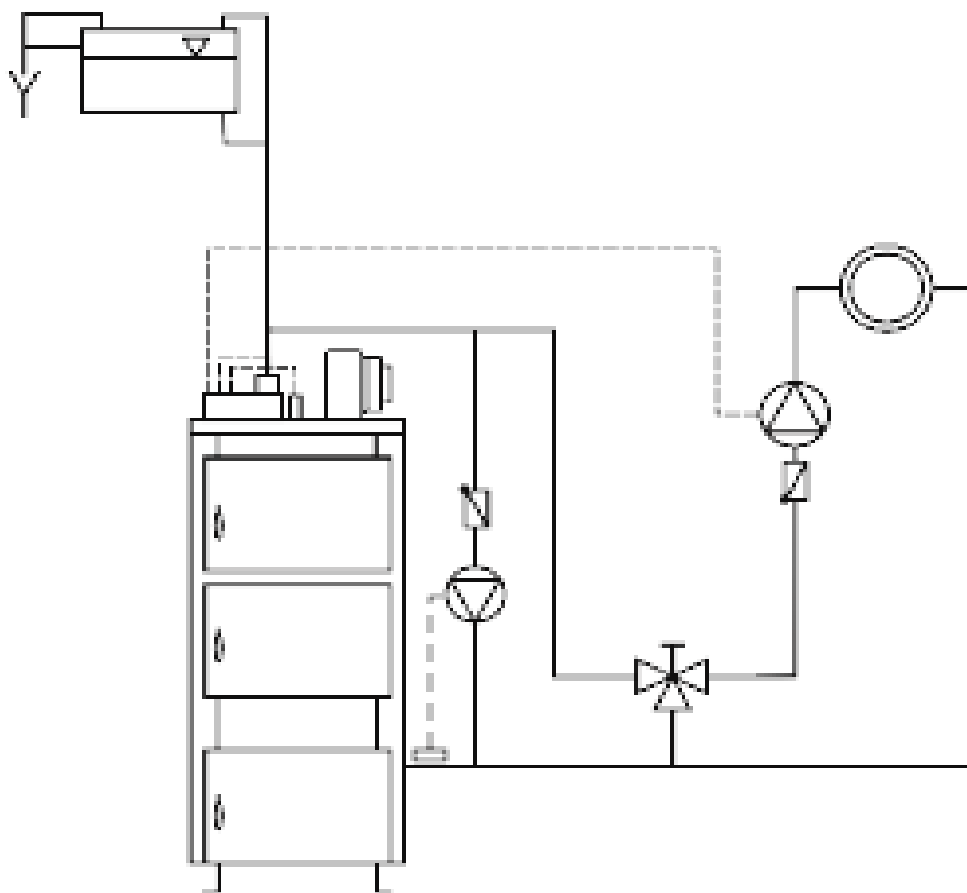
Рисунок 2 - Подключение с трехходовым клапаном
